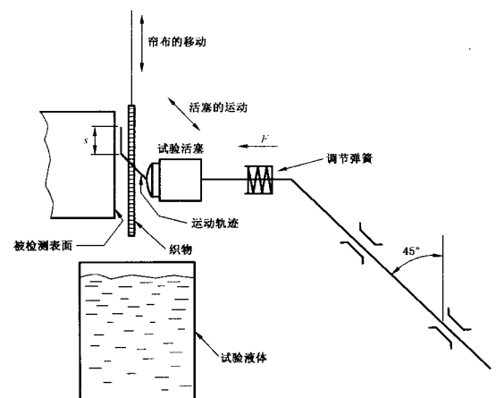
图 A.1 试验设备示意图(见 4.1)
