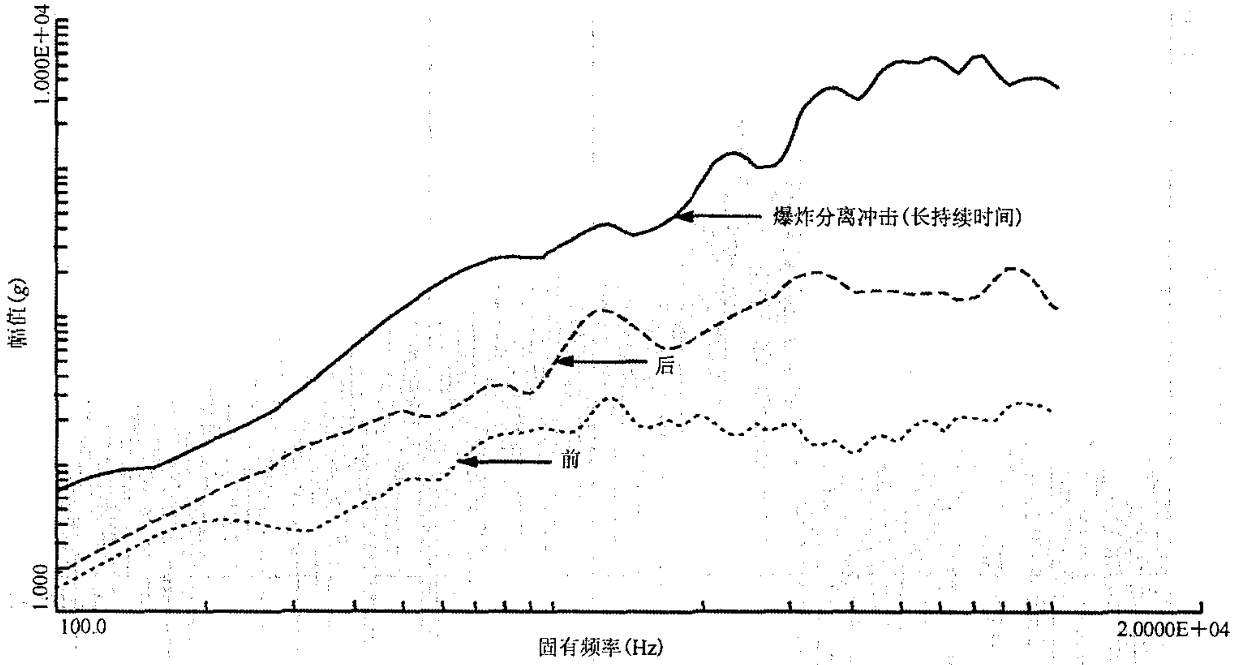
图 5 爆炸分离冲击及其之前和之后的最大绝对加速度冲击响应谱
